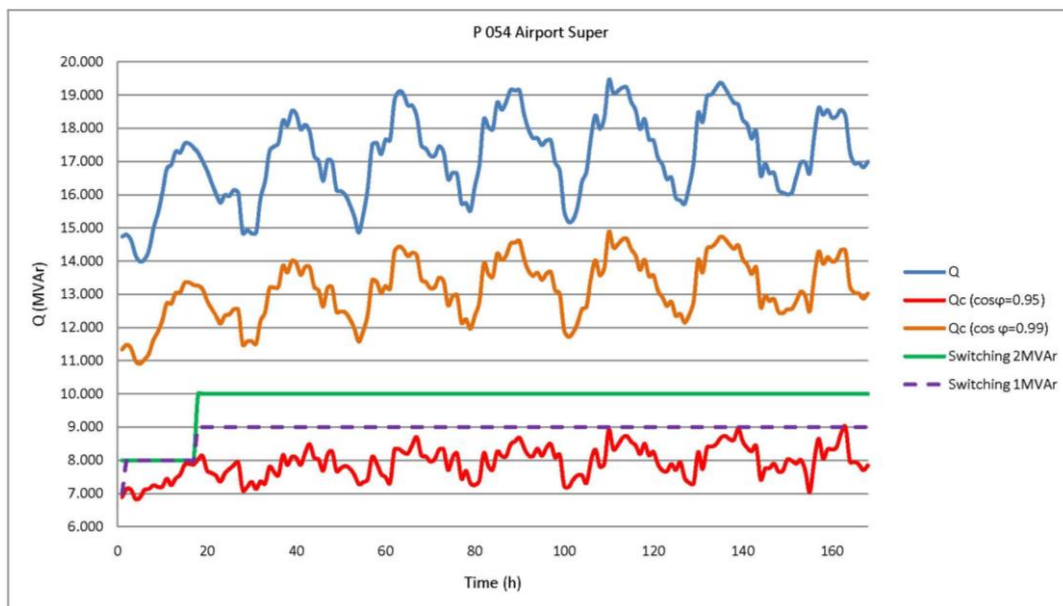
SLIKA 2 – REAKTIVNA SNAGA KOJU JE POTREBNO KOMPENZOVATI ZA POSTIZANJE \text{COS}\varphi=0,95-0,99 I DIJAGRAM SKLOPNIH OPERACIJA ZA REGULACIONE STEPENE OD 1 MVAR I 2MVAR U LETNJEM PERIODU
